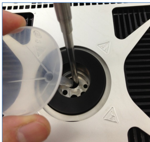
②付属のロートを用い、アルミナボールを注入。 *こぼれないようご注意ください。
