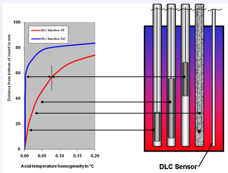
深さによる温度分布
