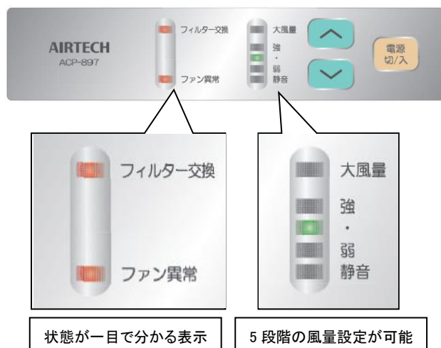
操作パネル
